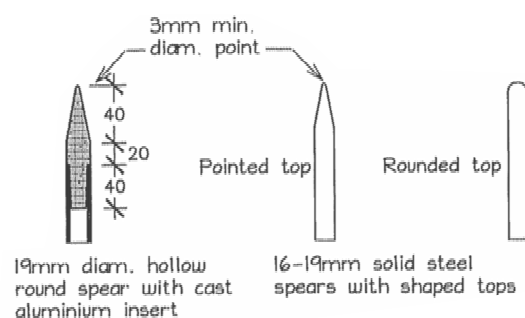
OPTIONAL SPEAR TOPS
